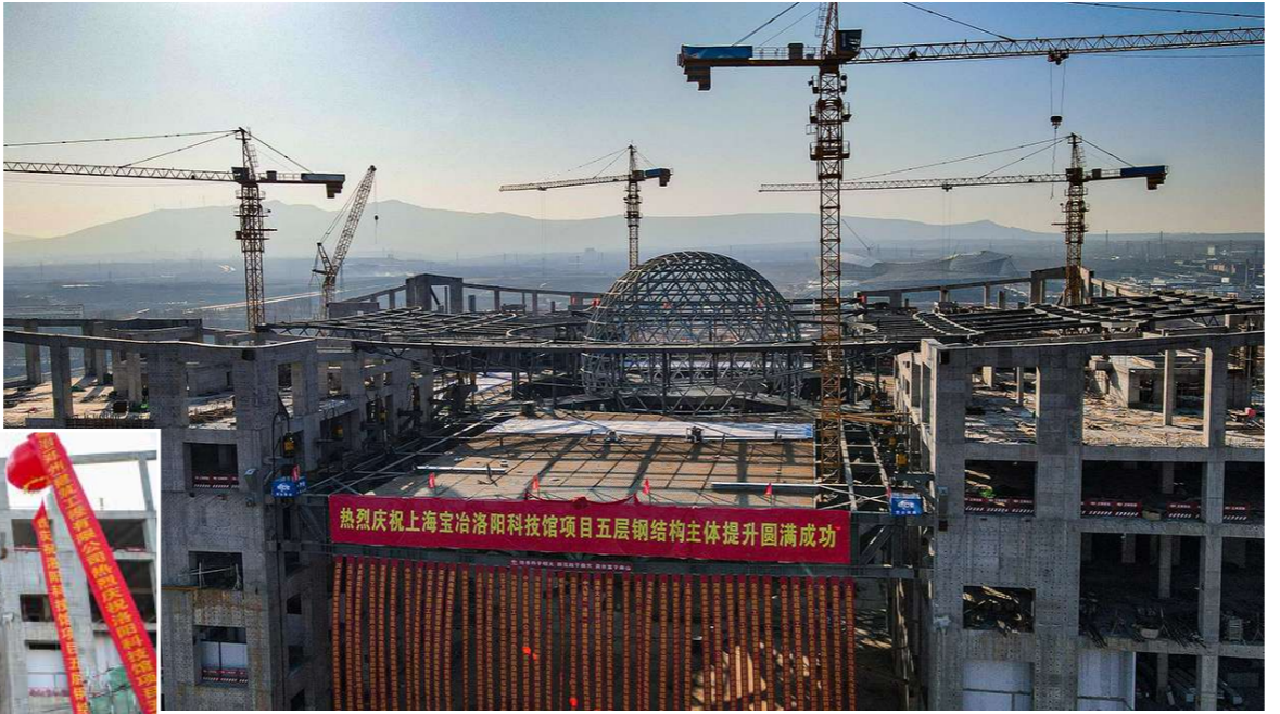
2021年12月20日,洛阳科技馆项目五层钢桁架整体提升合拢顺利完成,创造了“两个之最”!一个是目前华中地区钢结构提升重量之最,达到了6000t;一个是全国范围中心铝构球体直径最大,达到了33.23m。 该项目占地约162亩,项目总投资约21.34亿元,总建筑面积约11.85万平方米。规划设计地上五层,地下一层。项目于2020年10月启动建设,目前正按计划有序推进。(倪睿)
